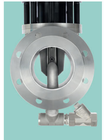
▲ Injektion direkt an den Mischflügeln.
